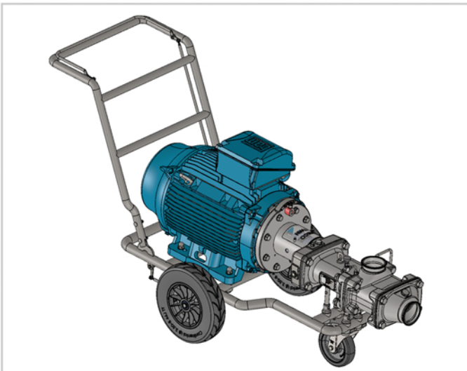
Frame 5 (Pumpcart)
